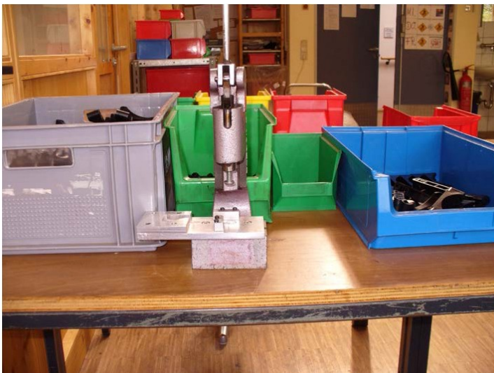
Abb. 2: In der Werkstatt für behinderte Menschen gliedert sich ein strukturierter Arbeitsplatz in den Aufgabenbereich (links), Arbeitsplatz (Mitte) und Fertigbereich (rechts)
